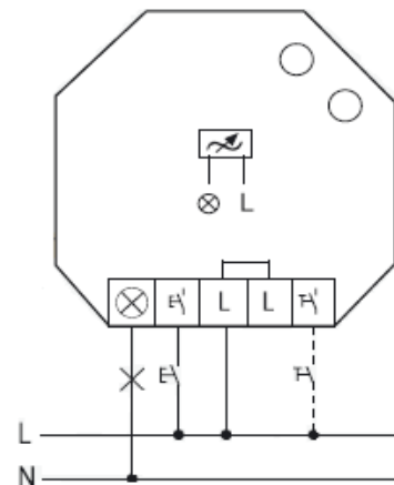
Koblingskjema
