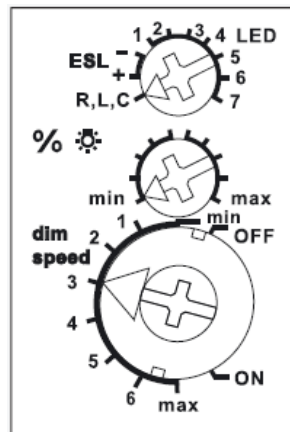
Funksjonsvelgere (Fabrikkinnstilling)
